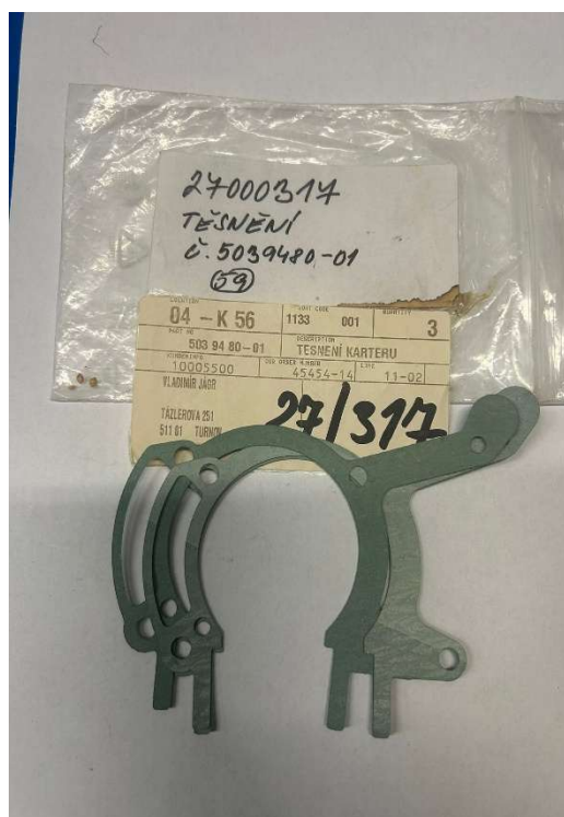
27000317 / Těsnění 5039480-01
